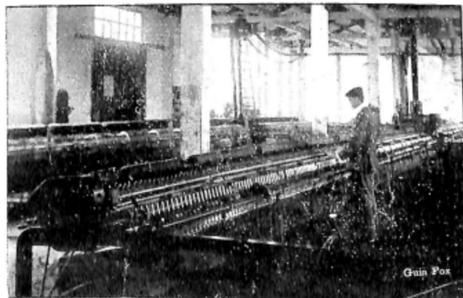
Outro aspecto da Secção de machinas da fabrica de tecidos de Chaves Irmão & C.
