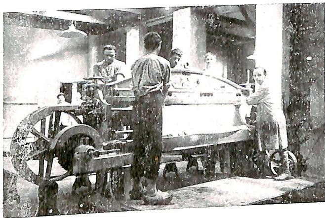
Machina para desdobrar o couro
