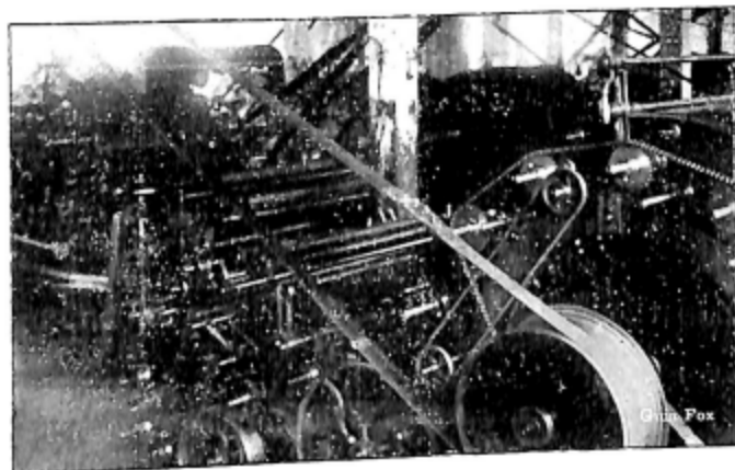
Um aspecto da carderia e outras machinas do estabelecimento fabril dos srs. Chaves Irmão & C.
