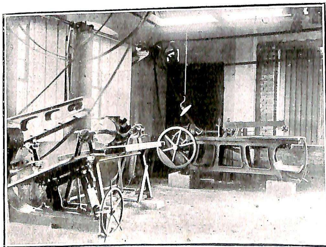
6.a secção. Parte da machinaria do Cortume Social Caxiense de Soares & C.
