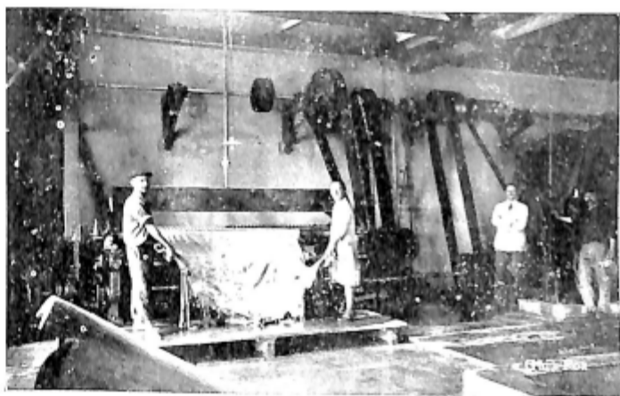
Machina descarnadora do couro
